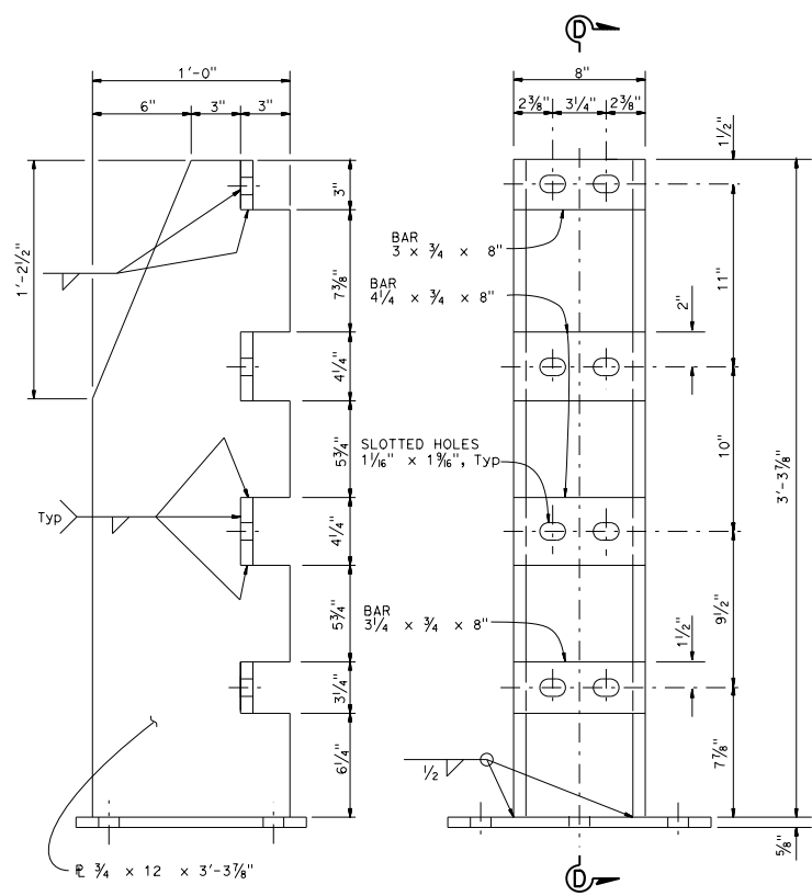
SECTION D-D
