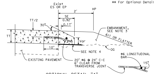
OPTIONAL DETAIL "A"
